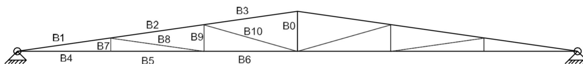
Figura 1: Numeração das barras da treliça.
