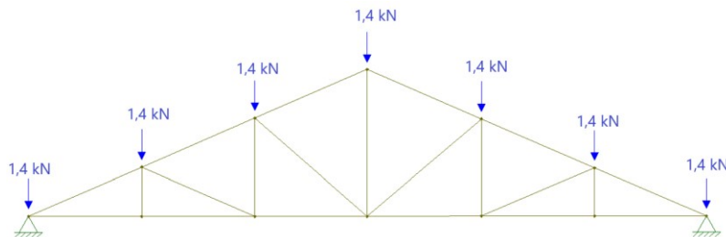
Figura 2: Modelo de cálculo da treliça.
