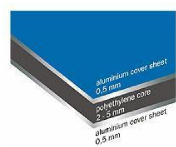
Figura 34: Corte esquemático da chapa de ACM.
