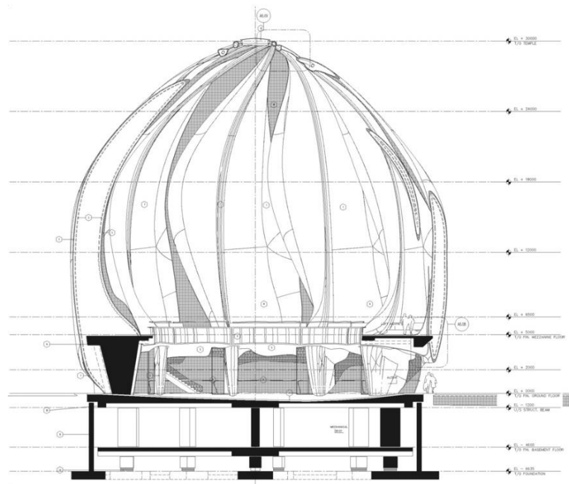
Figura 12: Corte do Templo Baha'i Fonte: < https://www.archdaily.com.br 22 >
