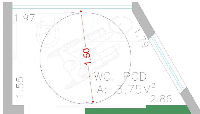
Figura 23: Banheiro PCD.
