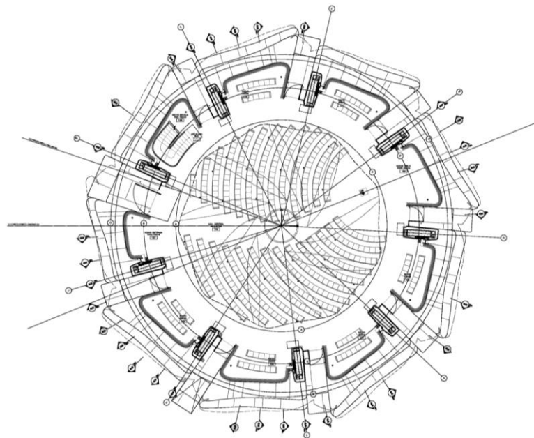
Figura 09: Planta baixa Térreo do Templo Baha'i
