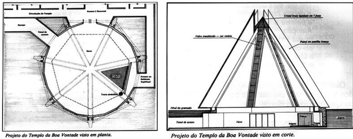
Figura 16: Planta baixa e corte do Templo da Boa Vontade.
