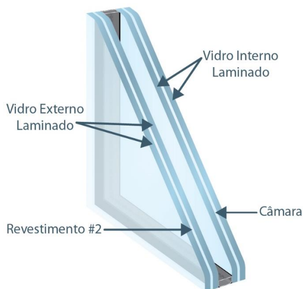
Figura 36: Corte esquemático do vidro.
