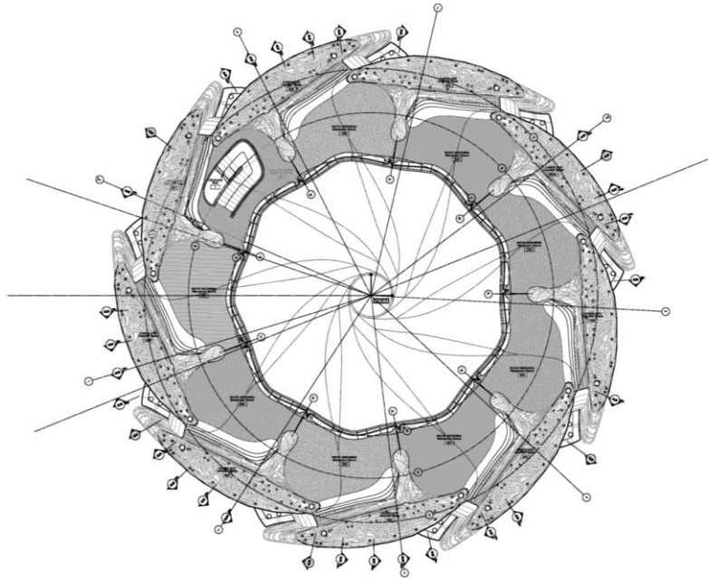
Figura 10: Planta baixa Mezanino do Templo Baha'i Fonte: < https://www.archdaily.com.br 20 >
