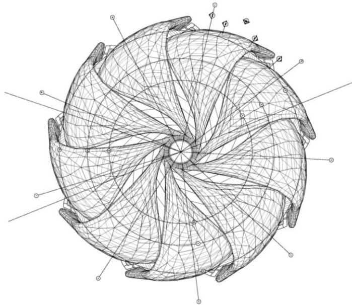
Figura 10: Planta baixa Mezanino do Templo Baha'i Fonte: < https://www.archdaily.com.br 20 >
