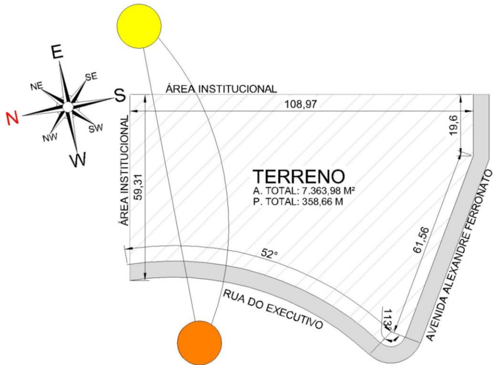
Figura 21: Orientação Solar.
