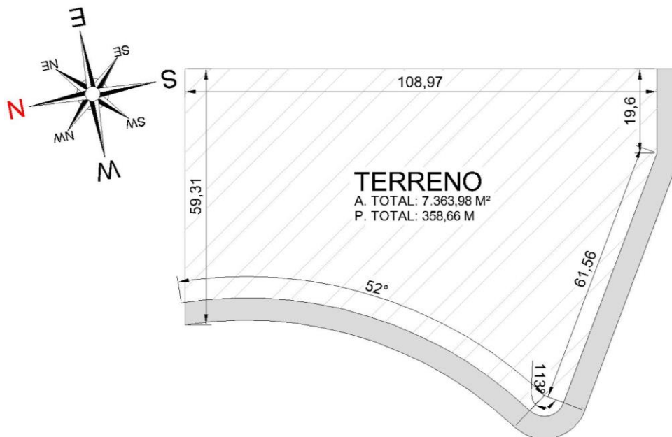
Figura 19: Dimensões do Terreno.
